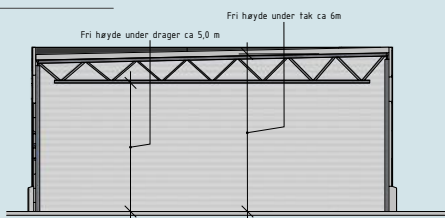
Snitt A-A
