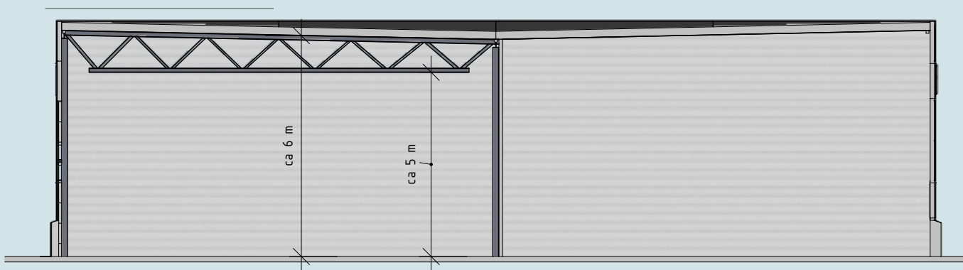
Snitt D:D
