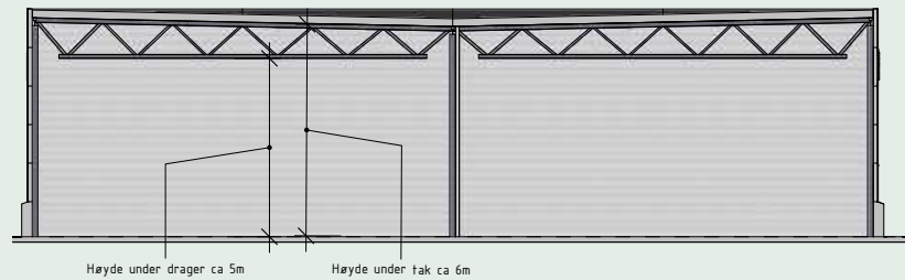
Snitt A-A
