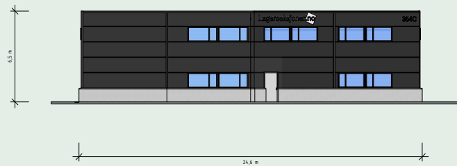
Fasade Nord-øst
